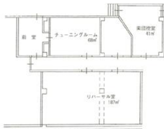
地 階
